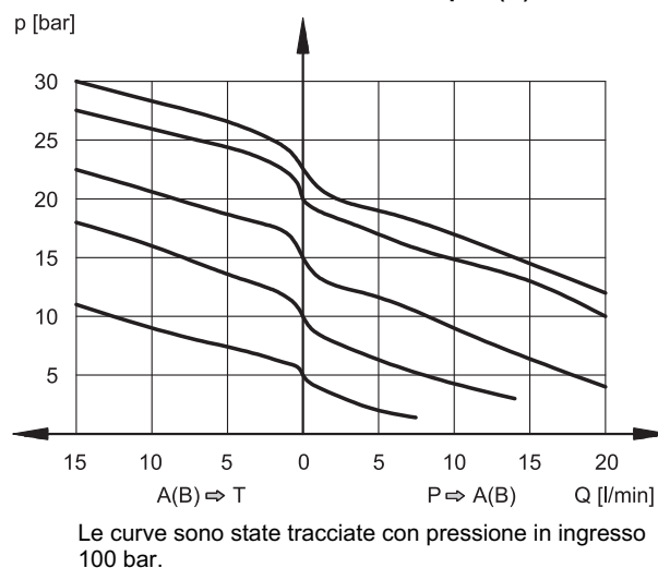
PERDITE DI CARICO \Delta p = f(Q)
